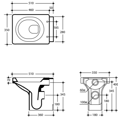
3518 vaso rettangolare unico scarico a parete "P" completo di curva tecnica per scarico scolo "S". rectangular wc pan wall outlet with waste pipe ?oor outlet
