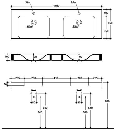
2 3536 lavabo 45x140 cm. doppia vasca sospeso, appoggio o su colonna monoforo One hole wall hung, free standing or on pedestal washbasin 45x140 cm double sink
